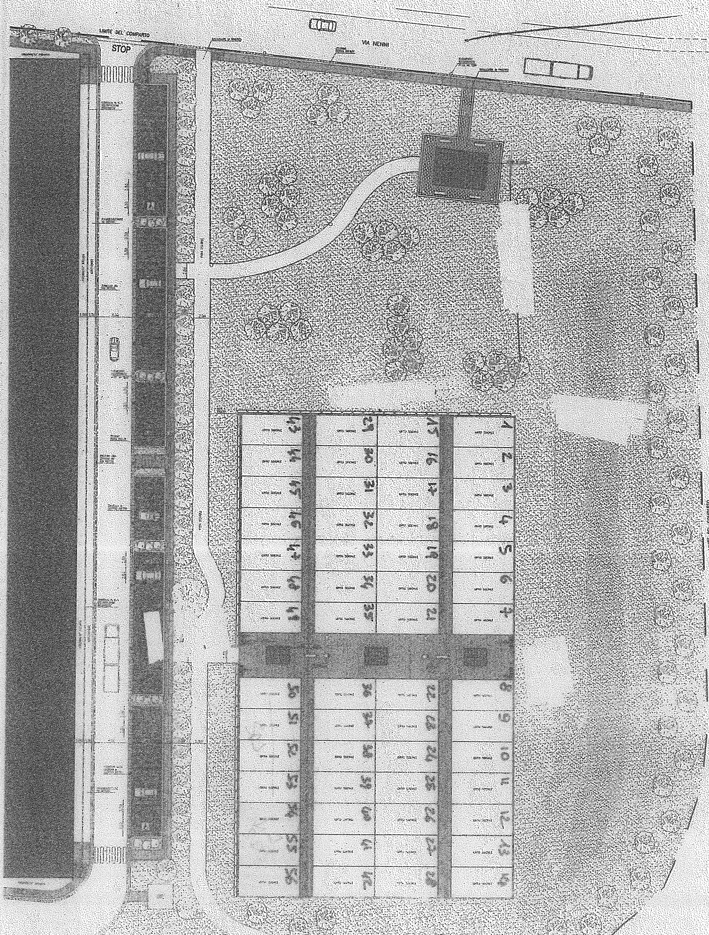
PLANIMETRIA GENERALE "AREA n. 11" SCALA 1:200
